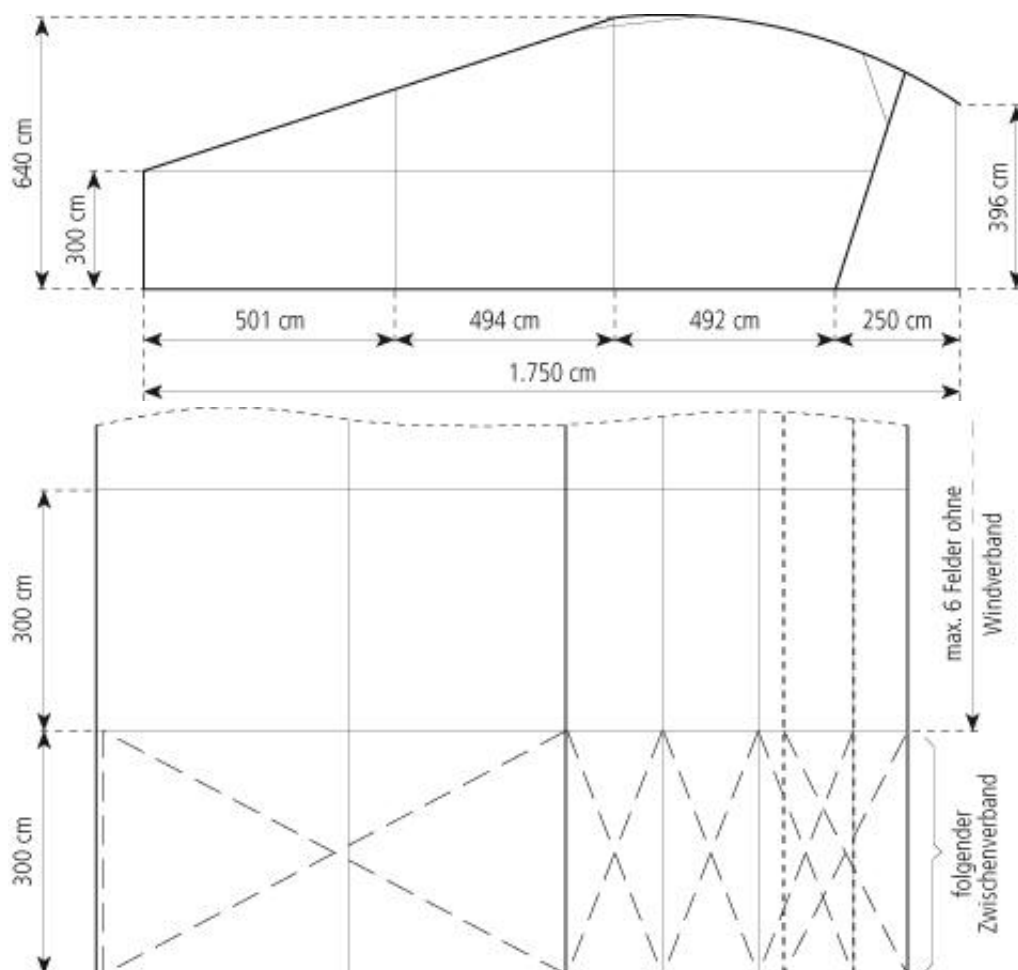
篷房俯视图与侧视图
