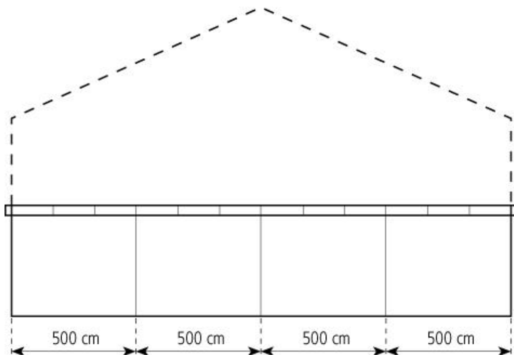
篷房俯视图与侧视图
