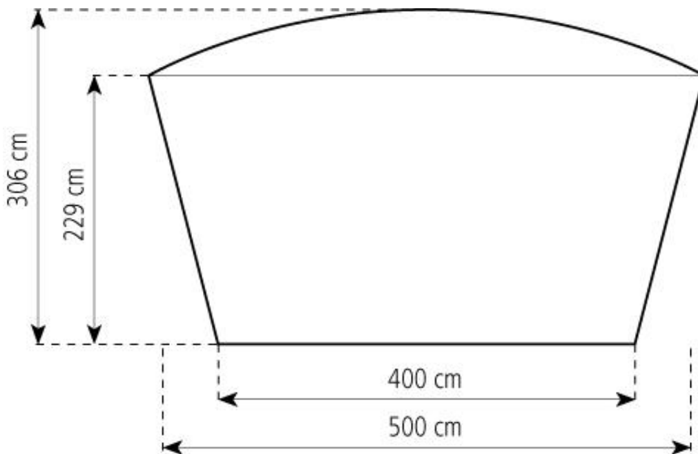
篷房俯视图与侧视图
