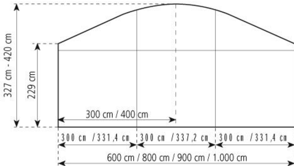
篷房俯视图与侧视图
