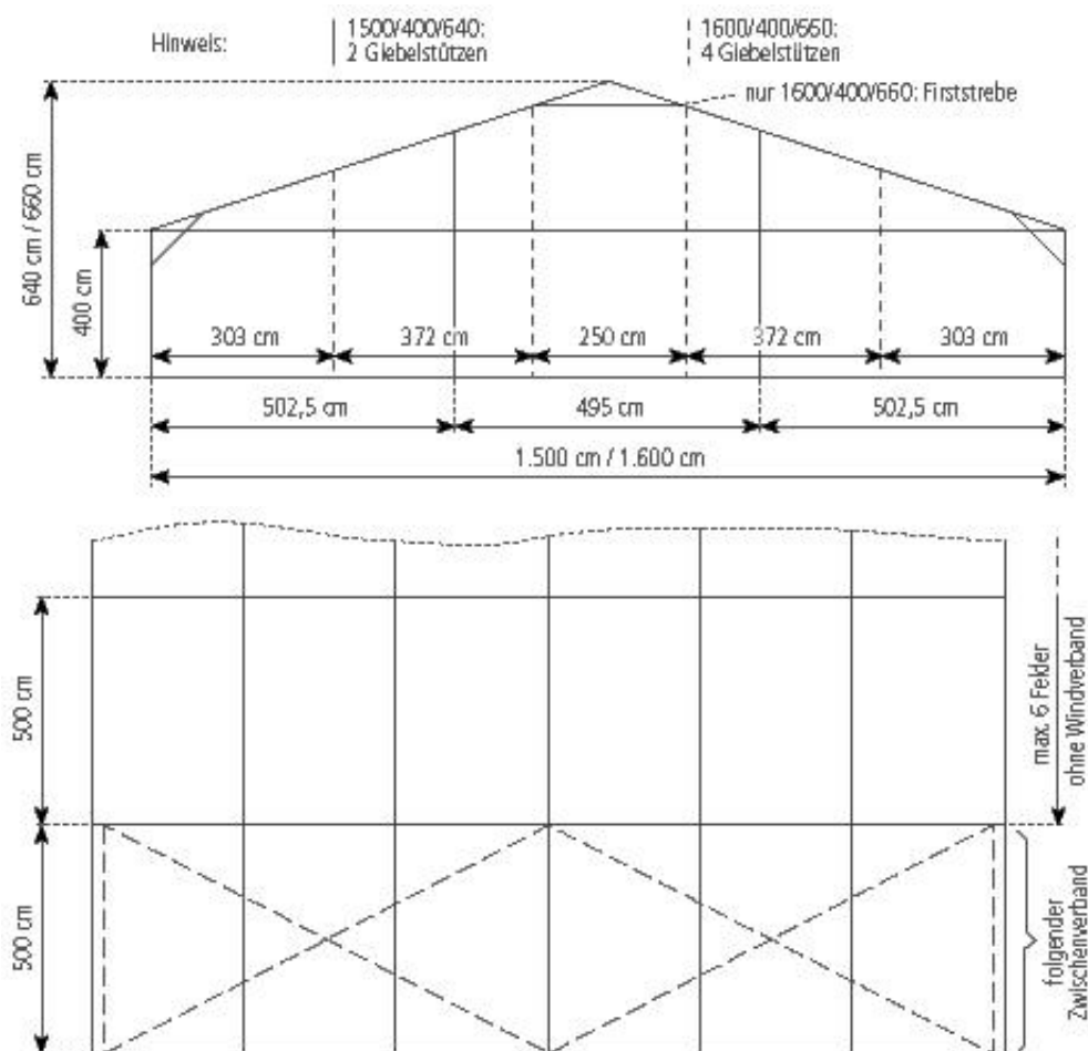
篷房俯视图与侧视图
